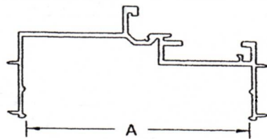
Delta Jamb
